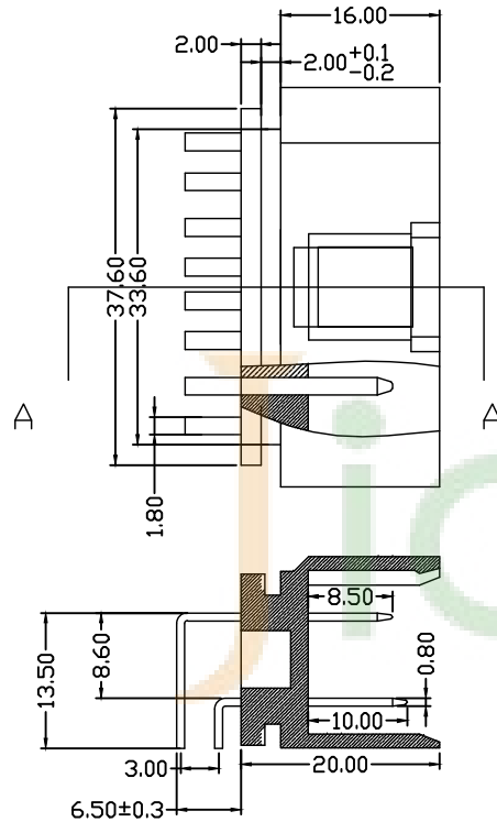
A-A Section
